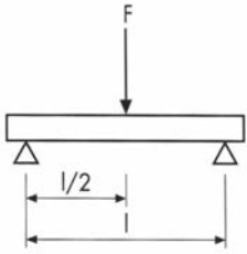
Схема нагружения 1
