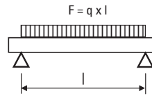
Схема нагружения 3
